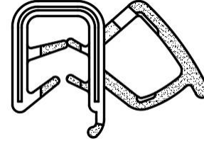
DOOR SEAL SLIDING F11077020
